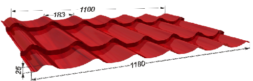
ЛСП «МОНТЕРРЕЙ» полезная ширина 1100 мм / габаритная ширина 1180 мм
