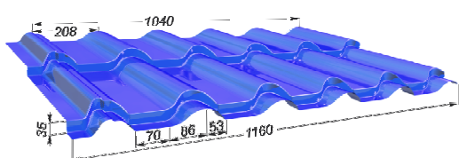
ЛСП «ДЮНА 35» полезная ширина 1040 мм / габаритная ширина 1160 мм
