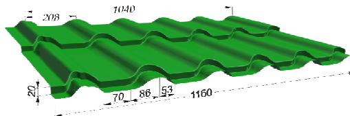
ЛСП «ДЮНА 20» полезная ширина 1040 мм / габаритная ширина 1160 мм
