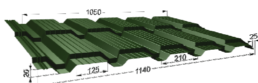
ЛСП «KASKAD» полезная ширина 1060 мм / габаритная ширина 1140 мм
