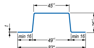
Стеновой обрешеточный профиль (СО)
