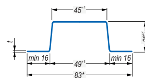
Стеновой обрешеточный профиль (СО)
